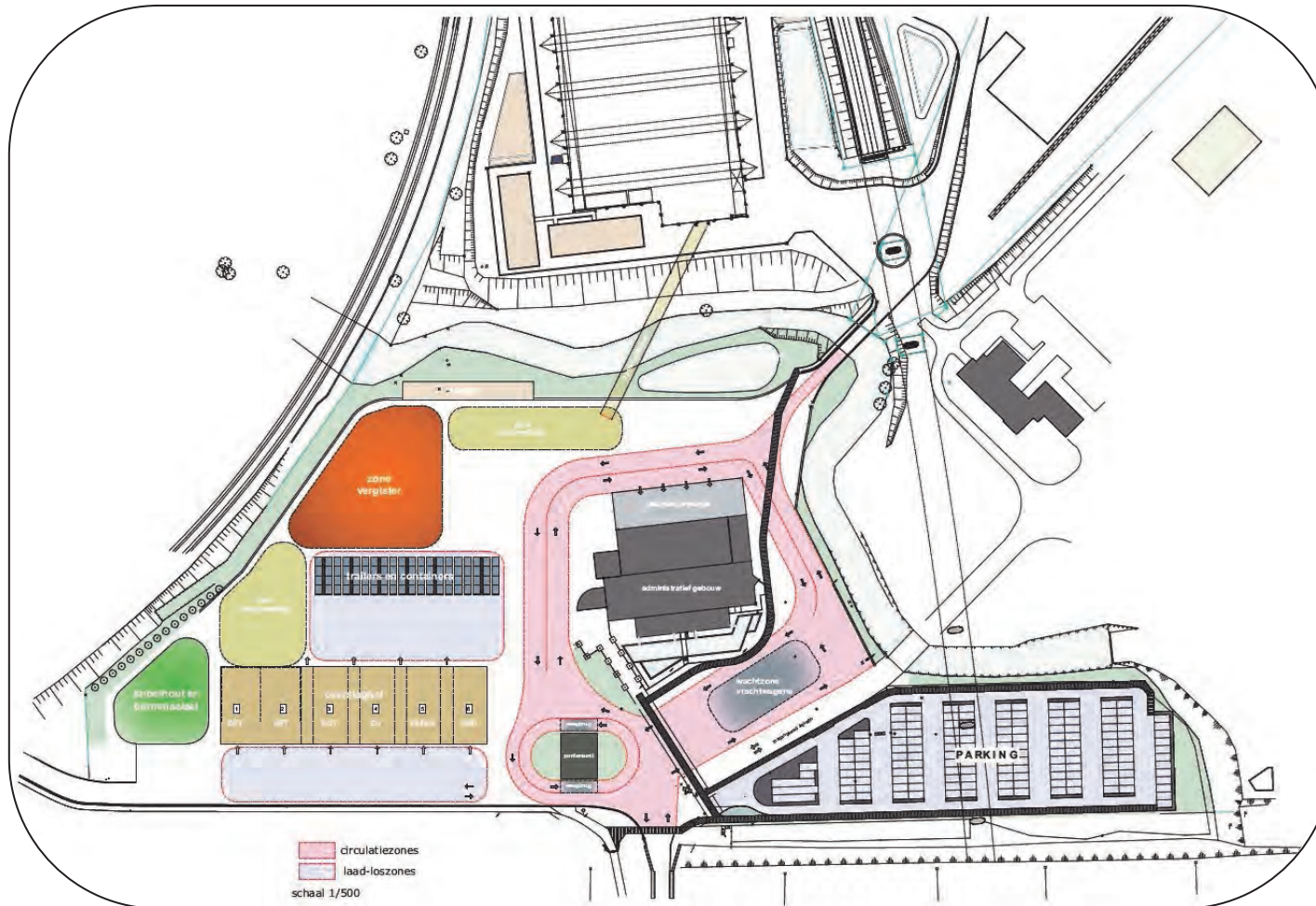
Masterplan EcoWerk-site met de vergistingsinstallatie, nieuwe stortbunkers, uitgebreide parking, aandacht voor veilige aan- en afvoer en optimale doorstroming van het verkeer op de site.
